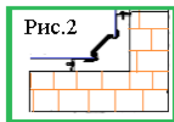
Рис.2 Угол объемный внутренний
